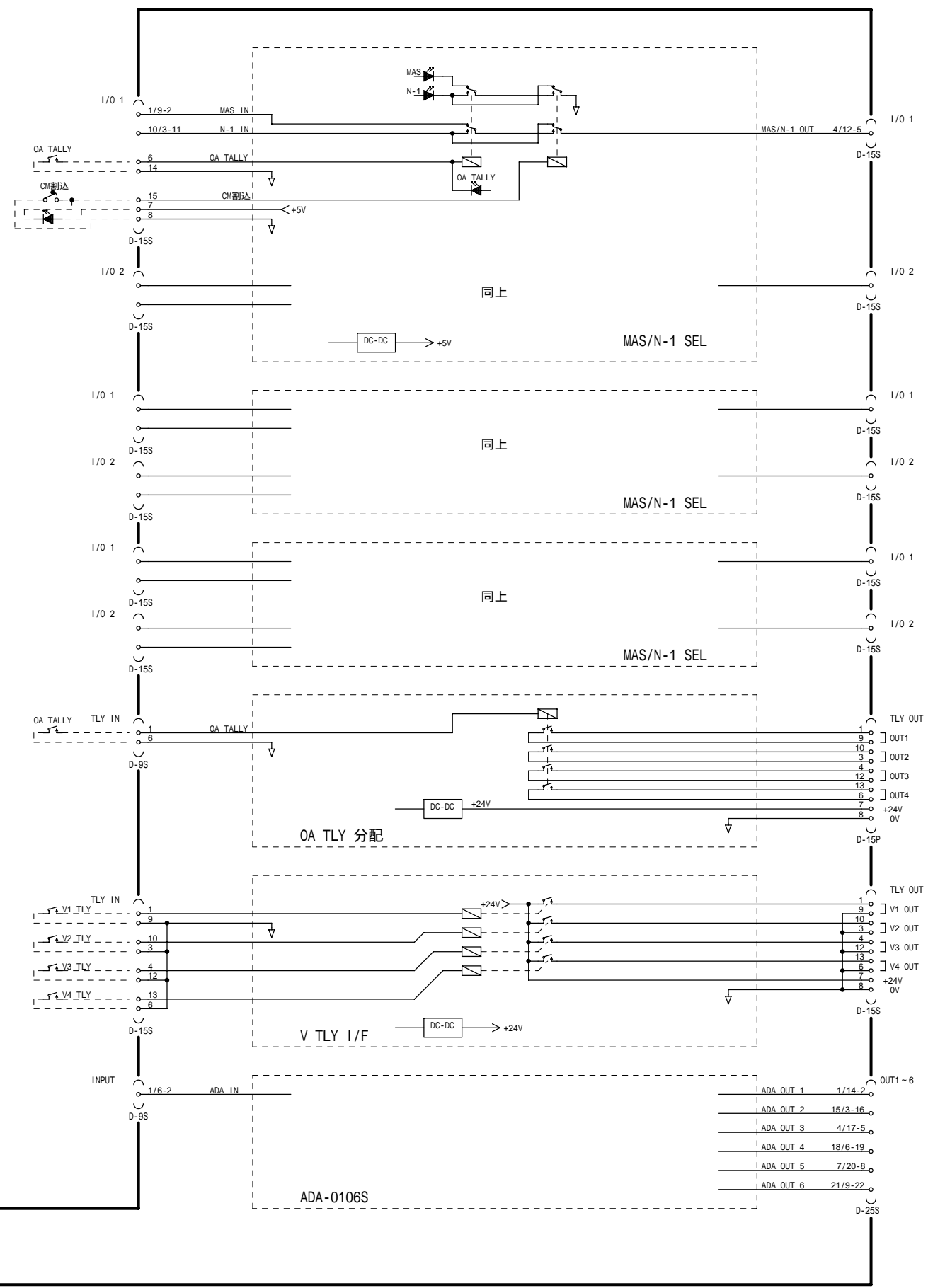
ユニット実装例
